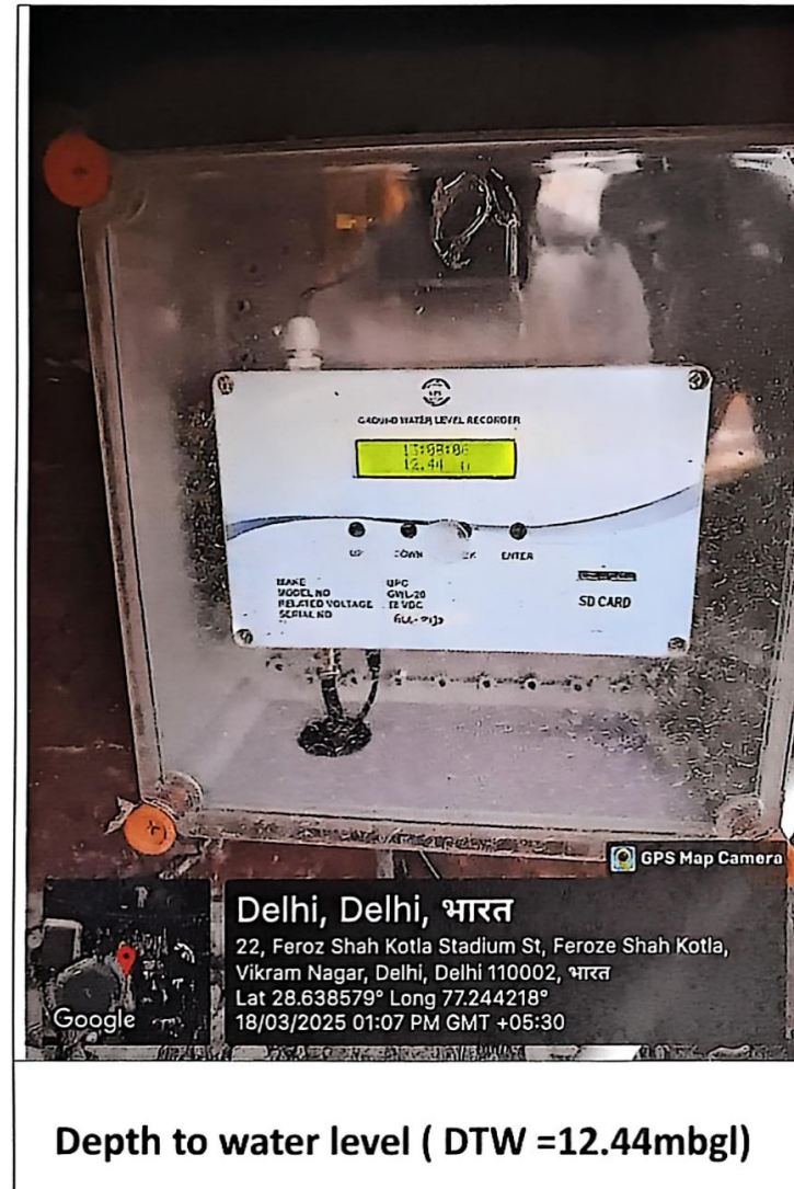
Piezometer
